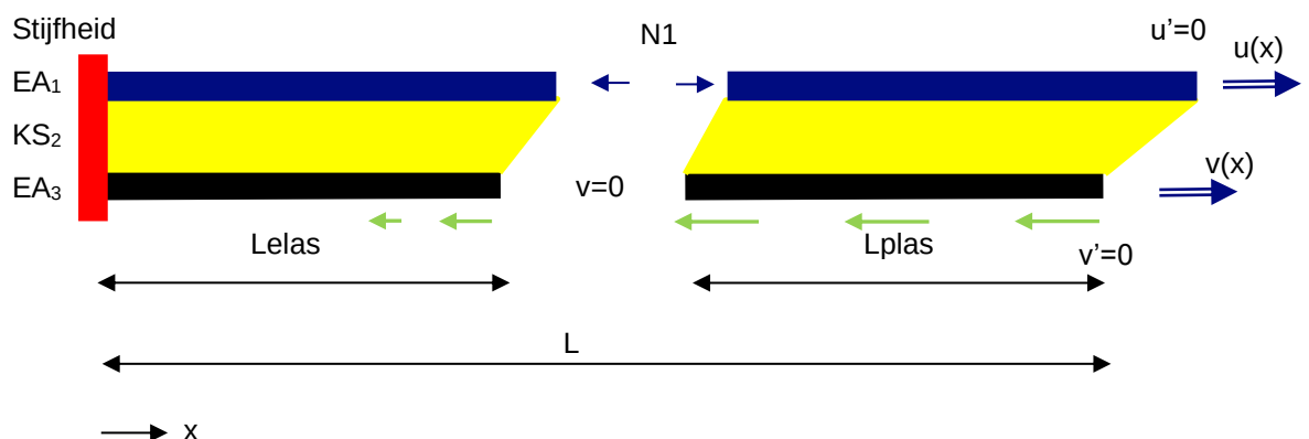
Figuur 14 Mechanica model opwarmen leiding
