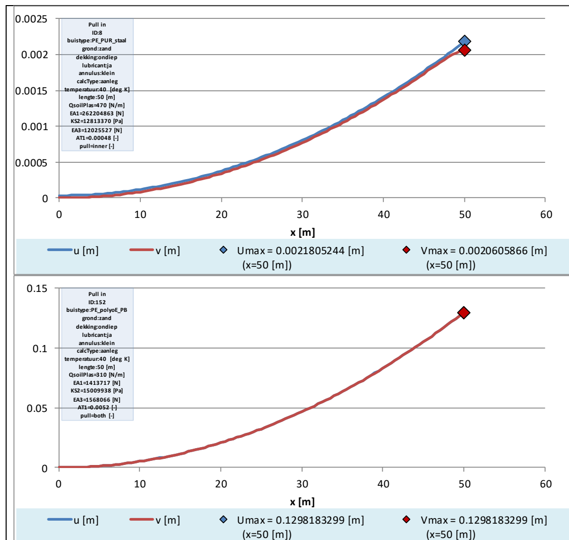
Figuur 11 Vervormingslijnen voor een trekkop die respectievelijk alleen de binnenbuis/beide buizen trekt
