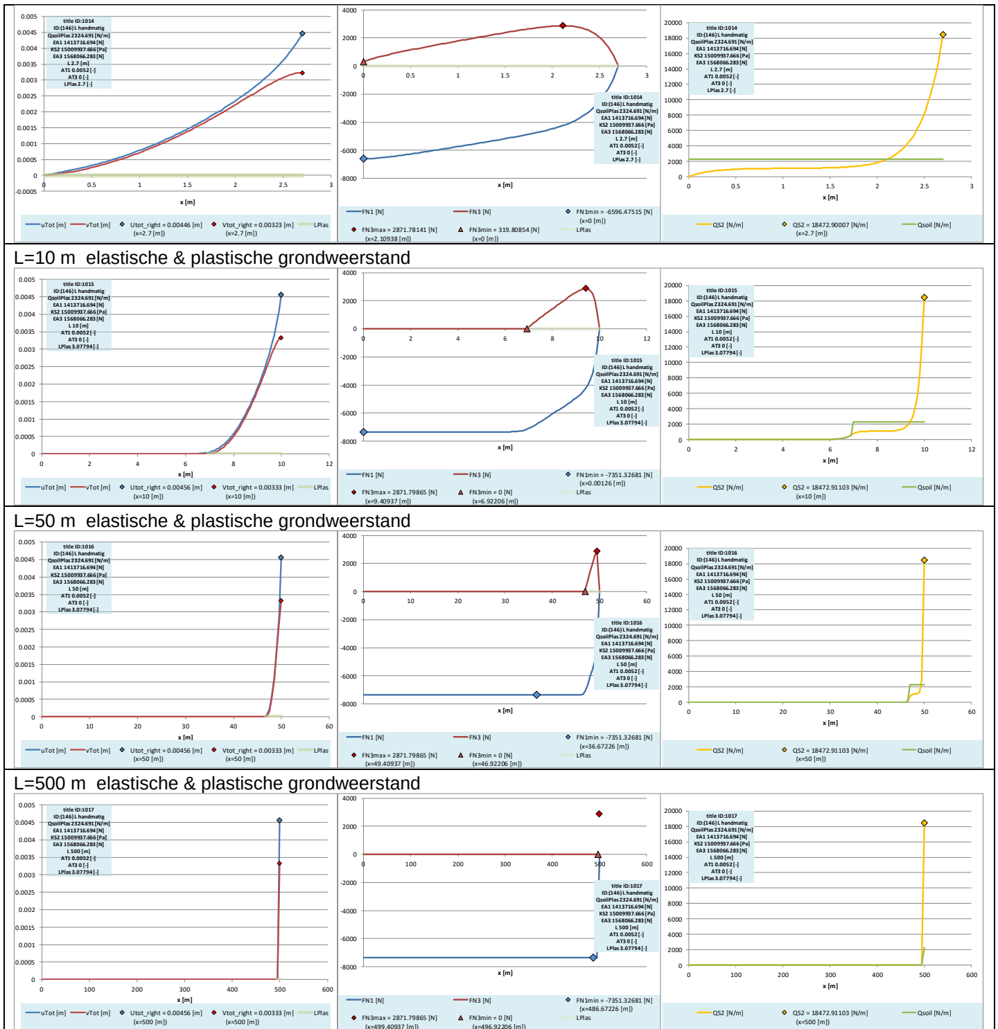
Figuur 30 Opwarmen variant ID=146, PE_polyoE_PE leiding; serie resultaten bij oplopende lengte
