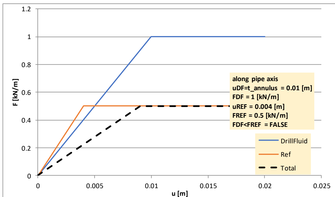
Figuur B4 Belasting evenwijdig aan leidingas
