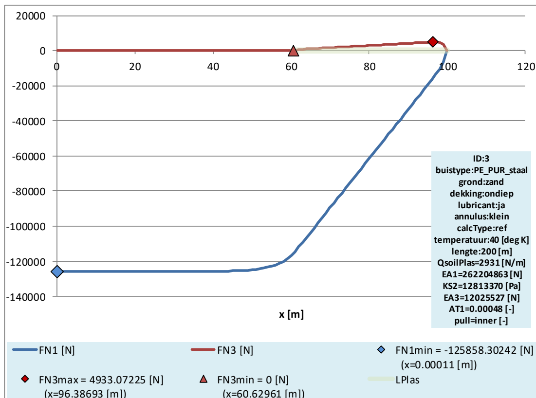
Figuur 16 Berekeningsresultaat opwarmen variant ID=3 normaalkrachten
