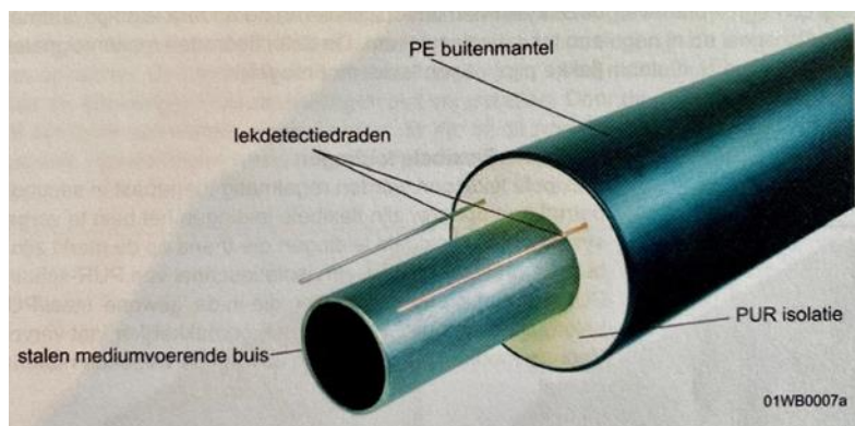
Figuur 1-1 Voorbeeld van een warmteleiding.
