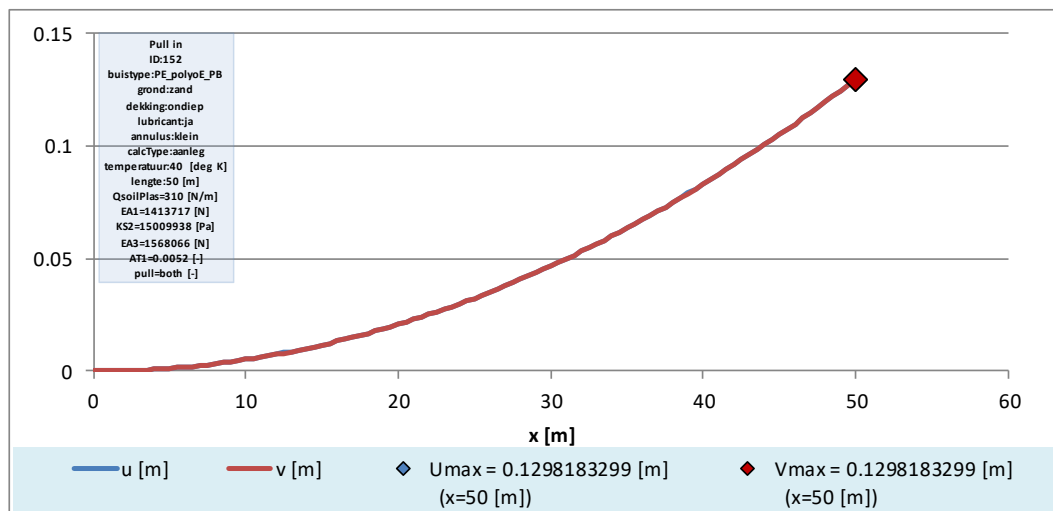
Figuur 22 Intrekken kunststof_PUR_kunststof (variant ID:152), blauwe lijn = binnenbuis, rode lijn = buitenbuis
