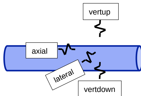
Figuur 4 Grondveren richtingen
